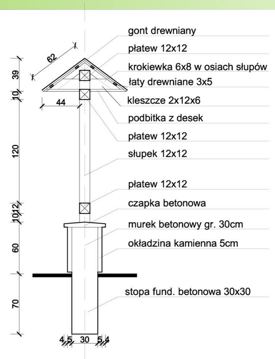
PRZEKRÓJ A-A , skala 1:25
