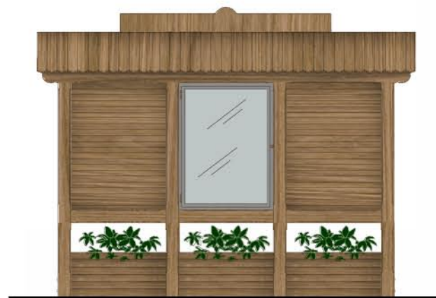
Element 2: 3D1, 3 pola, donice, 1 gablota skala 1:50
