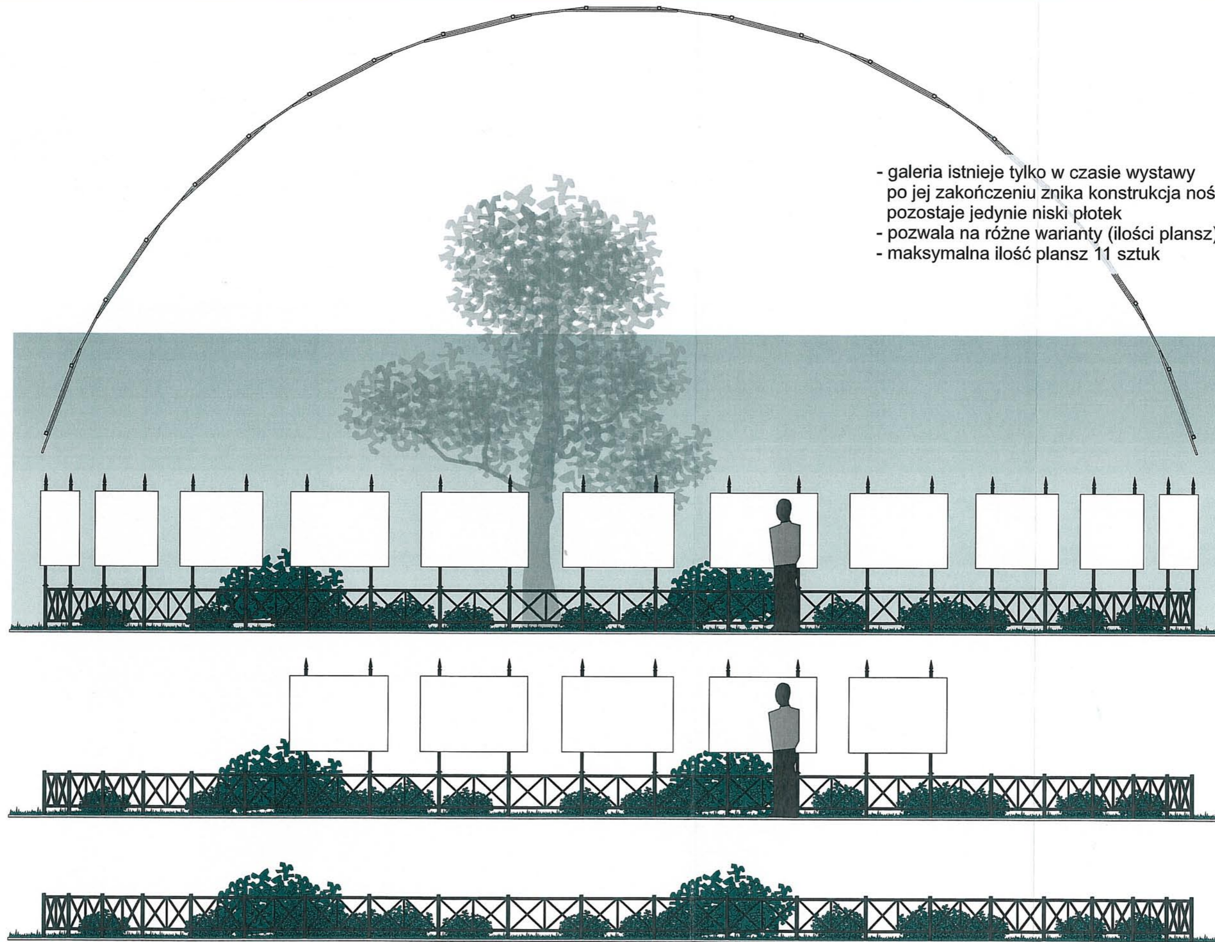
ELEMENT 1: TABLICE EKSPOZYCZYJE - UKŁAD TABLIC
